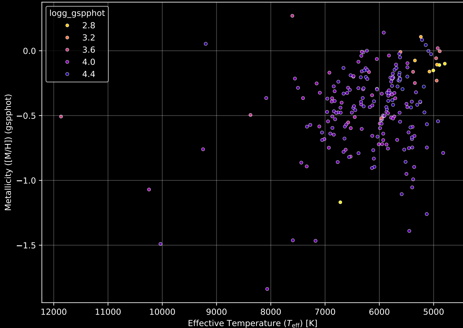
APOGEE DR17 Field: [CA_161-06_btx] Stellar Population Parameters (n= 220)
